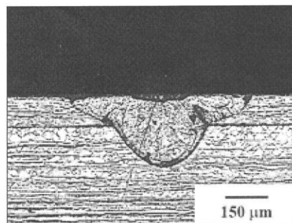
Figure 4. Secção transversal da amostra soldada.
