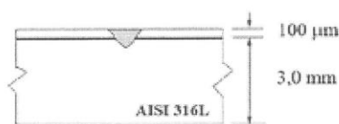
Figure 2. Desenho esquemático da junta soldada.
