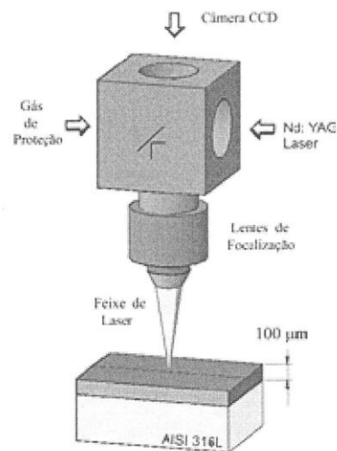
Figura 1. Diagrama esquemático do sistema de soldagem por laser pulsado de Nd:YAG
