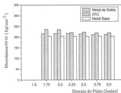
Figura 8. Perfil de microdureza Vickers do metal base, ZAC e metal de solda do aço AISI 316L em função da energia do pulso.
