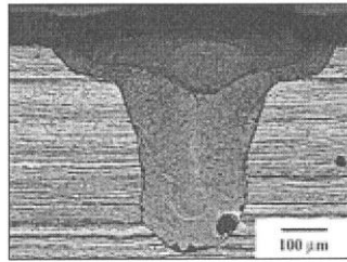
Figura 5. Secção transversal das juntas soldadas com laser pulsado de Nd:YAG com diferentes energias de pulso (Ep). a) 1,5 J, b) 2,0 J, c) 2,25 J, d) 2,5 J, e) 2,75 J, f) 3,0 J.
