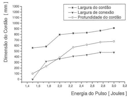
Figura 6. Relação entre a energia do pulso [Ep] e a geometria do cordão.
