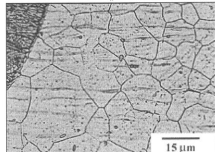
Figura 7. Microestrutura típica da zona de fusão (a) e da ZAC (b) do aço AISI 316L. (amostra soldada com 2.0 Joules).
