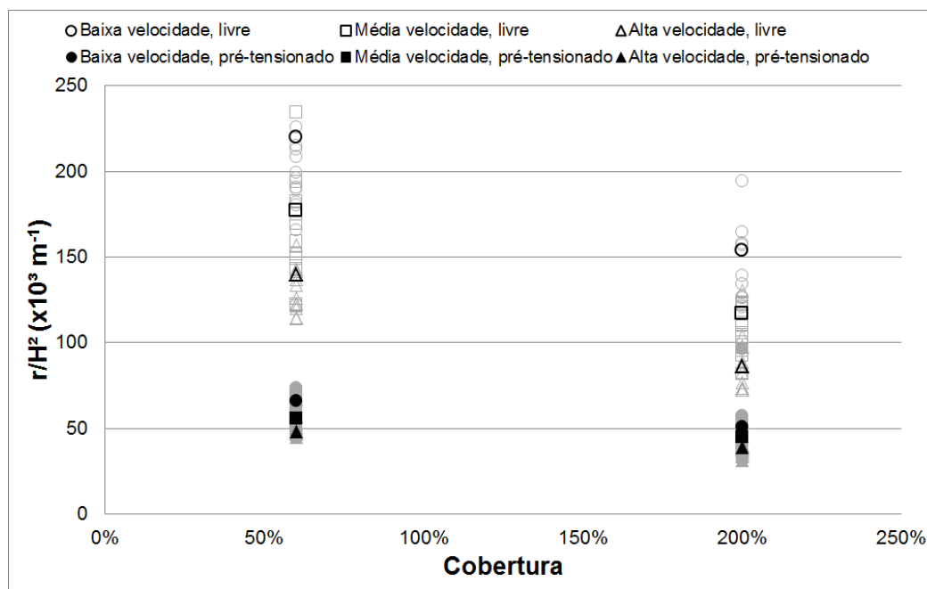
Figura 9. Efeito da cobertura sobre r/H^2 . Chapas jateadas com granalha S550. Em destaque: dados fictícios calculados para chapa de 7mm.
