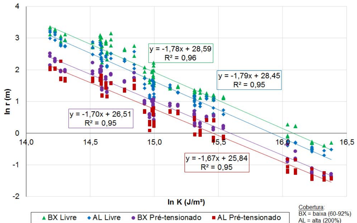
Figura 7. Relação semi-empírica entre densidade de energia cinética e raio de curvatura dos CPs conformados por jateamento com granalhas.
