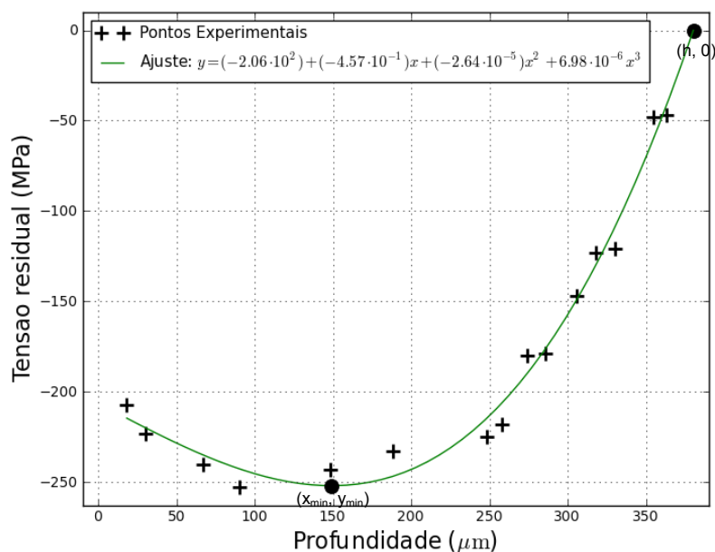
Figura 5. Perfil de tensões residuais após JCG em chapa da liga 7050, 2 mm de espessura, granalha S230, velocidade baixa, sem pré-tensão.
