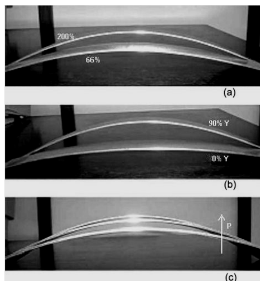
Figura 1. Efeitos das variáveis de jateamento no empenamento dos corpos de prova da liga 7050, espessura 2 mm. (a) Diferentes coberturas (66% e 200%); (b) Diferentes pré-tensioamentos (0 e 90% do limite de escoamento); (c) Diferentes pressões do jato (20 psi, 40 psi e 60 psi).
