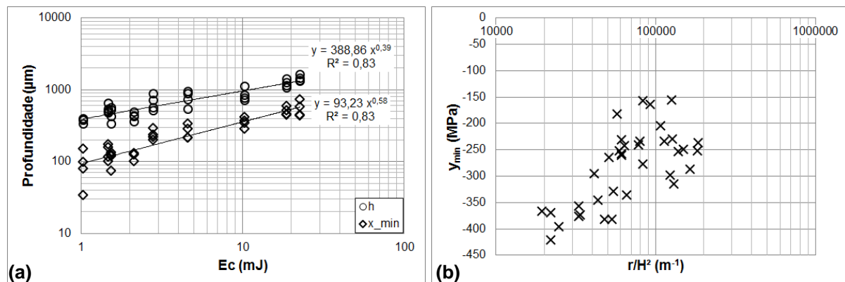
Figura 8. Relações entre (a) profundidade da máxima compressão e da espessura da camada deformada e a energia cinética das granalhas; (b) máxima compressão e o raio de curvatura normalizado.
