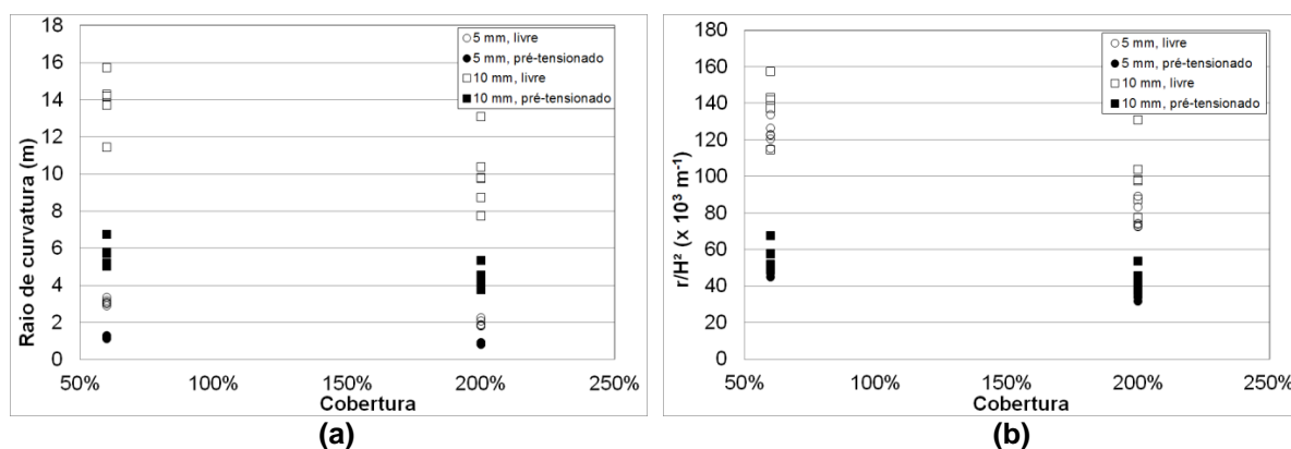
Figura 6. Efeito da cobertura em chapas de 5 mm e 10 mm, jateadas com granalha S550, 30 psi, sobre: (a) Raio de curvatura ( r ); (b) Raio de curvatura normalizado ( r/H^2 ).
