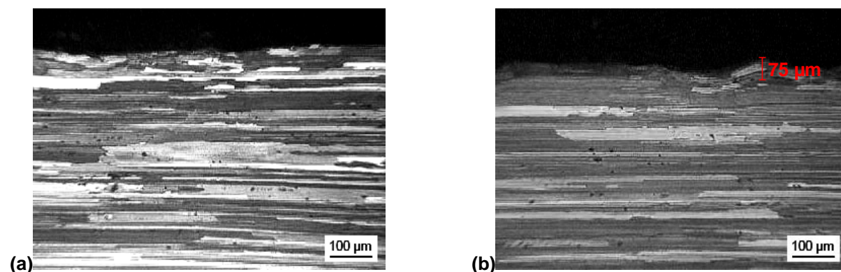
Figura 3. Camada de grãos recristalizados na liga 7475. (a) Após 30 min; (b) Após 60 min.
