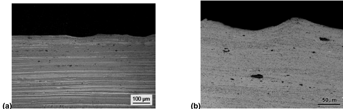
Figura 2. Microestrutura das amostras jateadas, próximas às endentações na superfície. (a) Liga 7050, ataque Barker; (b) Liga 7475, ataque Keller.
