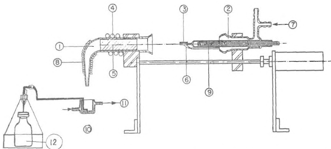
FIGURA 1. Esquema do equipamento: 1. Tubo externo de quartzo (fixo). 2. Tubo interno de quartzo (móvel). 3. Suporte de platina com óxido de telúrio. 4. Forno de indução. 5. Tubo de platina \varnothing = 22 mm. 6. Termopar. 7. Fluxo de \text{O}_2 = 30-40 ml/min. 8. Aquecimento. 9. Resistência elétrica. 10. Solução de NaOH. 11. Circulação de água de refrigeração. 12. Frasco coletor.
