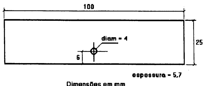
Figura 1. Dimensões do corpo-de-prova
