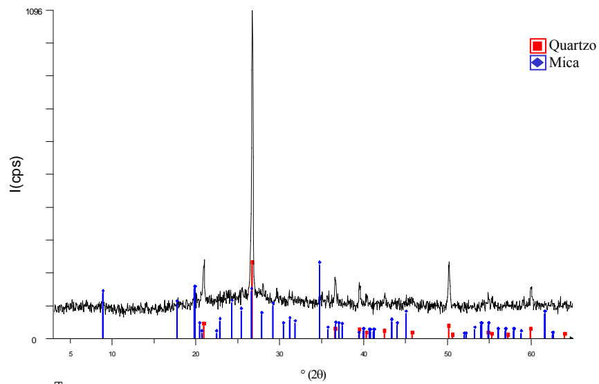
Figura 2. Gráfico de DRX de uma amostra Marajó
