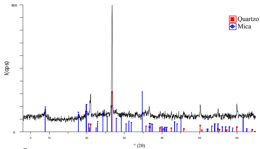
Figura 3. Gráfico de DRX de uma amostra contemporânea.
