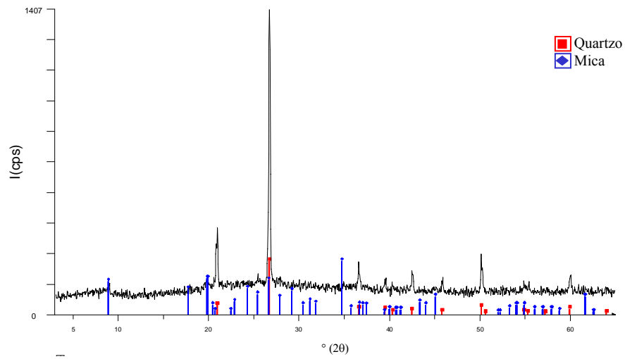
Figura 1. Gráfico de DRX de uma amostra MAE
