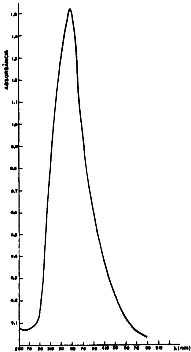
FIGURA 4 - Espectro de absorção na região do visível do bis-[N-benzoil-N-fenilhidroxilamato] Cobre II submetido a radiação \gamma de uma fonte de Cobalto-60 ( 3,0 \times 10^5 Gy)
