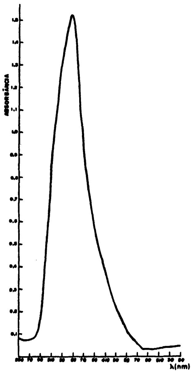
FIGURA 2 - Espectro de absorção na região do visível do bis-[N-Benzoyl-N-phenylhydroxylamine] Cobre II
