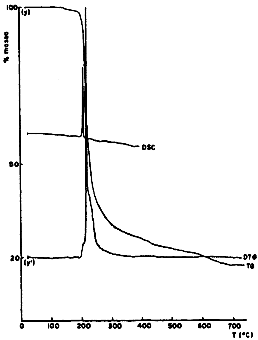
FIGURA 3 - Curvas TG, DTG e DSC do bis-[N-benzil-fenilhidrocloridinato] Cobre (II)
