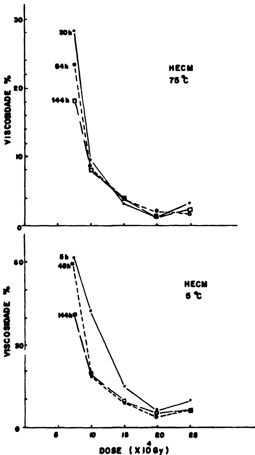
Fig. 4 - Viscosidade % em função da dose de radiação e do tempo após a irradiação a duas temperaturas, de amostras de 1% de HECM.
