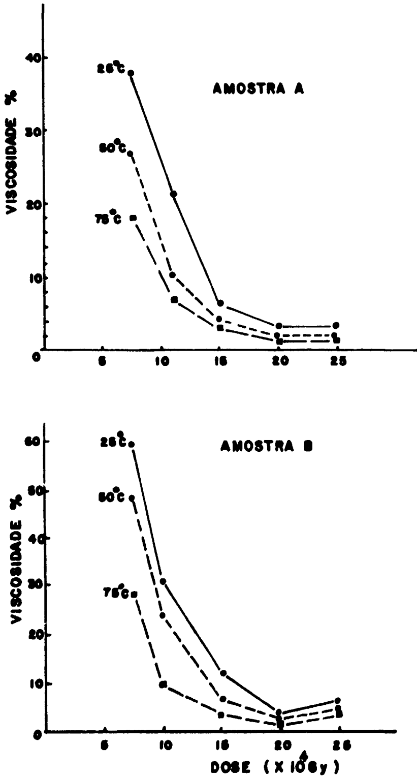
Fig. 2 Viscosidade % em função de dose de radiação e de temperatura de 1% HECM.
