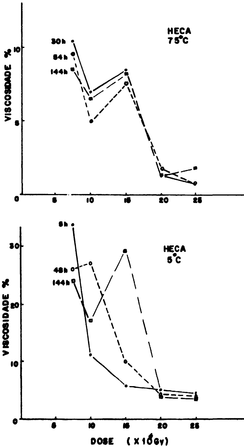
Fig. 3 - Viscosidade % em função da dose de radiação e do tempo após irradiação a duas temperaturas de amostras de 1% HECA.
