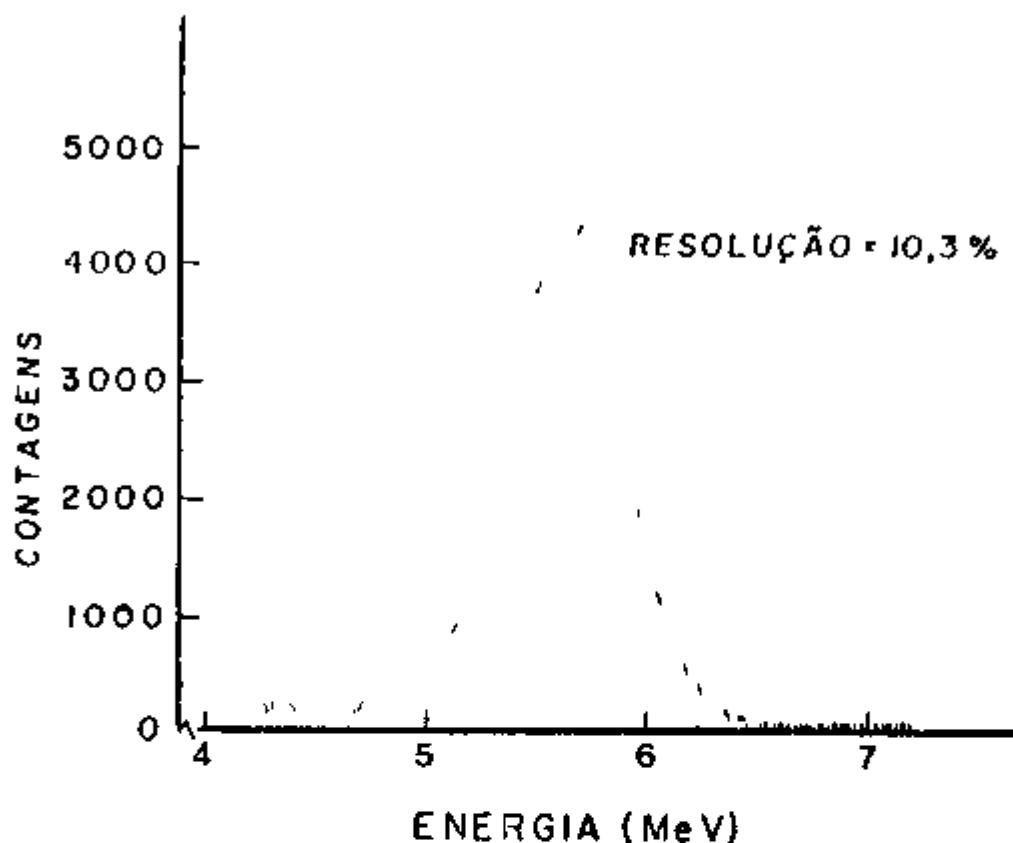
Figura 2 - Espectro da Radiação Alfa do ^{241}\text{Am}
