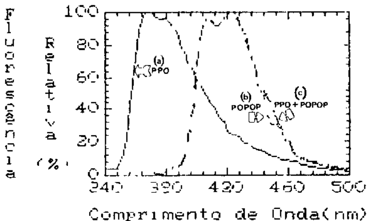
Figura 1 - Espectros de Fluorescência de uma Amostra do Plástico Cintilador
