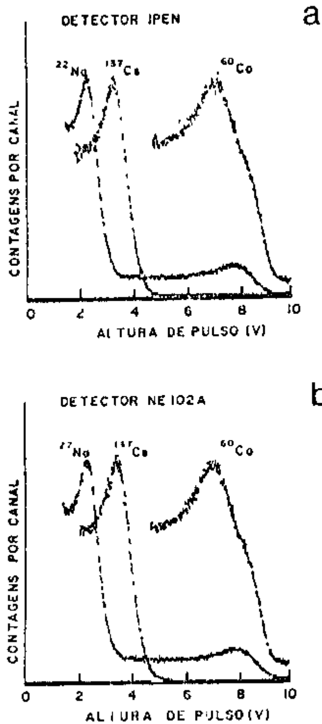
Figura 3 - Análise de Altura de pulso entre a) o detector confeccionado no IPEN b) o detector NE 102A da Nuclear Enterprises
