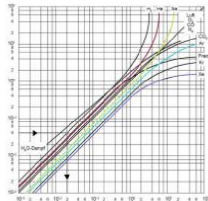
Figura 6. Curvas de conversão para a leitura realizada num ambiente diferente do Nitrogênio.
