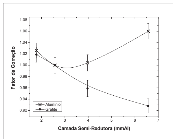
Figura 3. Dependência energética das câmaras de ionização para as qualidades de radiação RQR. Os fatores de correção foram normalizados para a qualidade RQR5.
