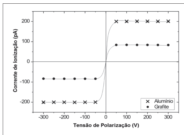
Figura 1. Curvas de saturação para as câmaras com eletrodos coletores de Alumínio e Grafite (RQR 5).
