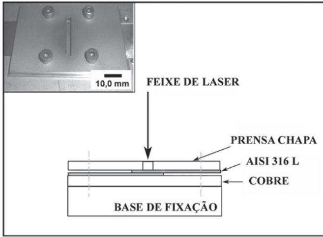
Figura 2. Esquema do dispositivo de fixação das amostras de lâmina fina.
