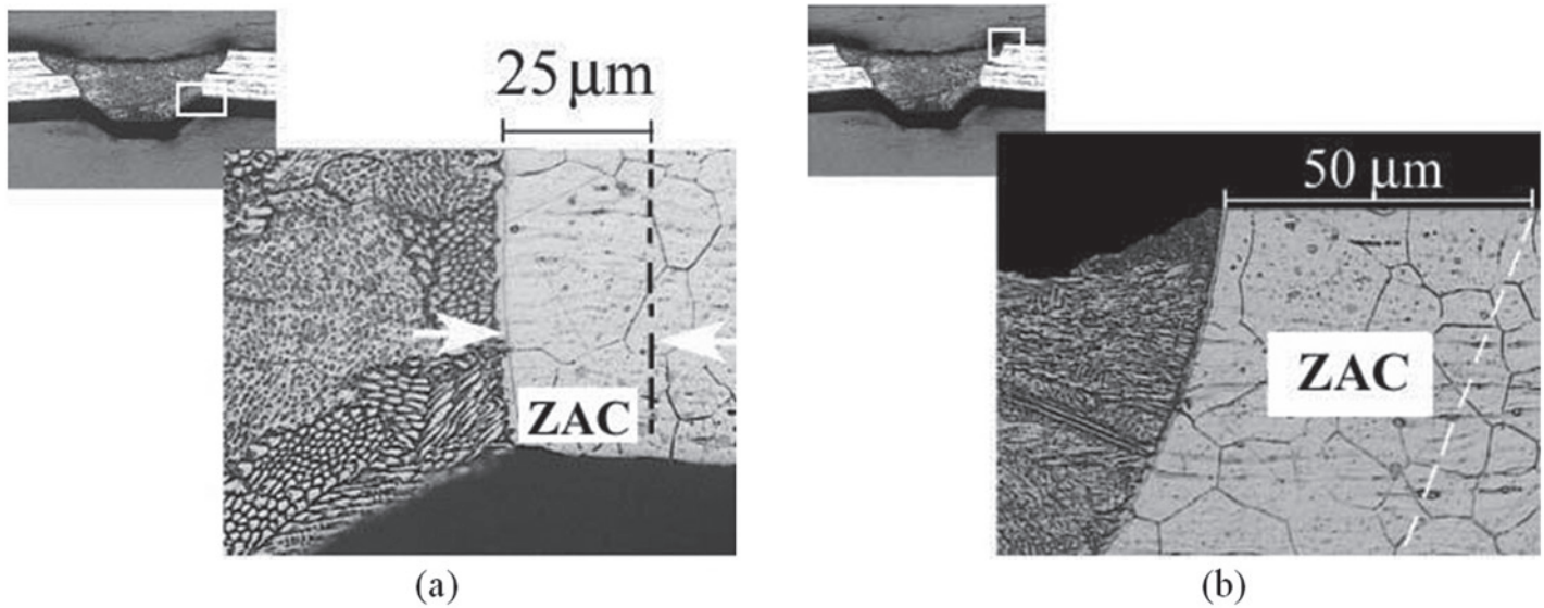
Figura 8. Zona afetada pelo calor na lâmina superior (a) e na lâmina inferior (b) da junta. (amostra soldada com 2,25 Joules).
