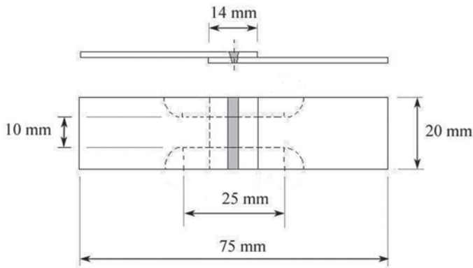
Figura 3. Configuração da junta para extração dos corpos de prova.
