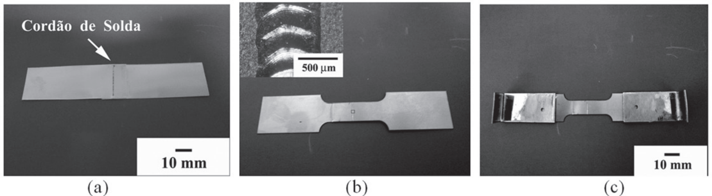
Figura 5. Amostra soldada (a), cortada (b) e preparada para ensaio de tração (c).
