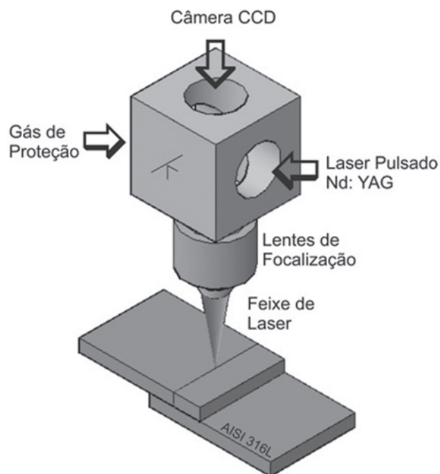
Figura 1. Diagrama esquemático do sistema de soldagem por laser pulsado de Nd:YAG
