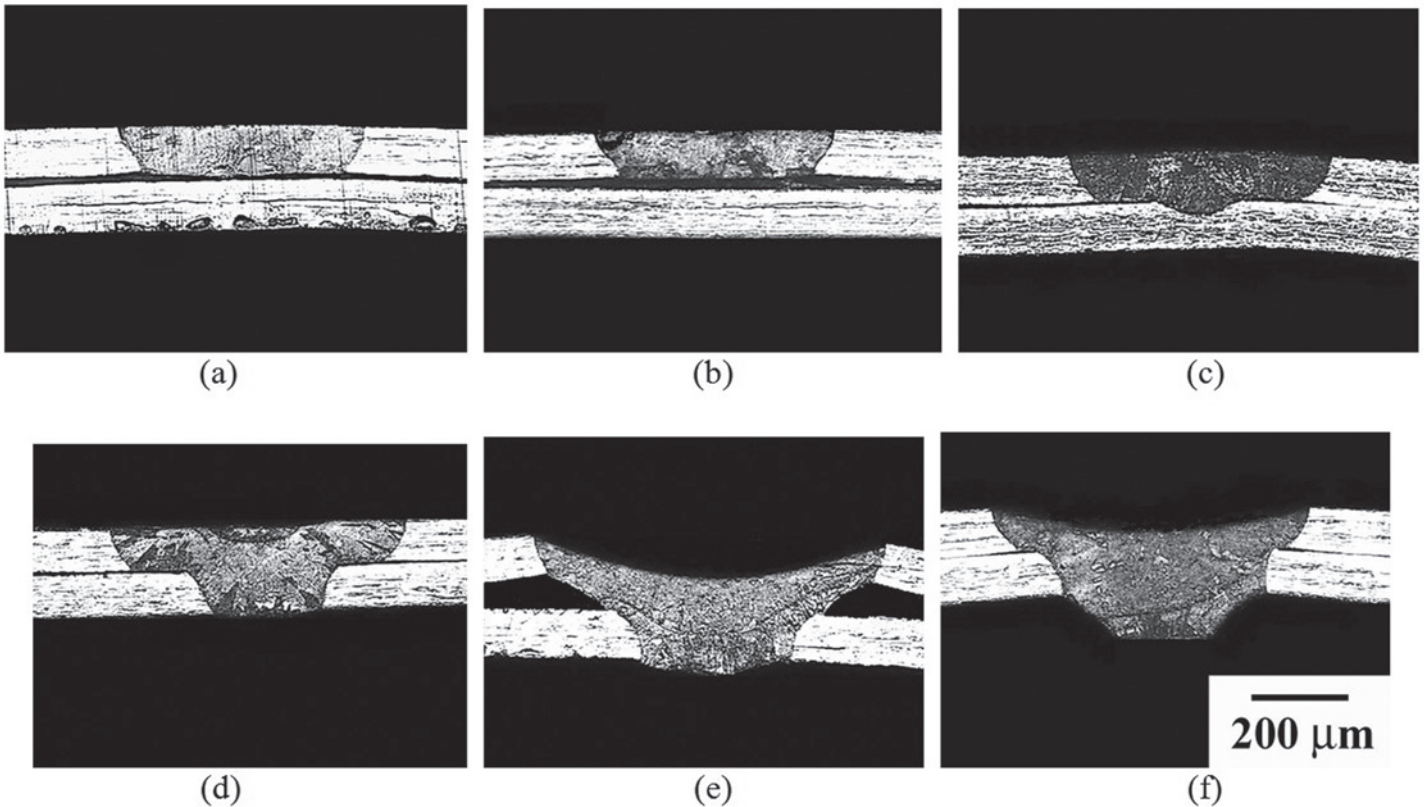
Figura 6. Seção transversal das juntas soldadas com laser pulsado de Nd:YAG com diferentes energias de pulso ( E_p ). a) 1,0 J, b) 1,25 J, c) 1,50 J, d) 1,75 J, e) 2,0 J e f) 2,25 J.
