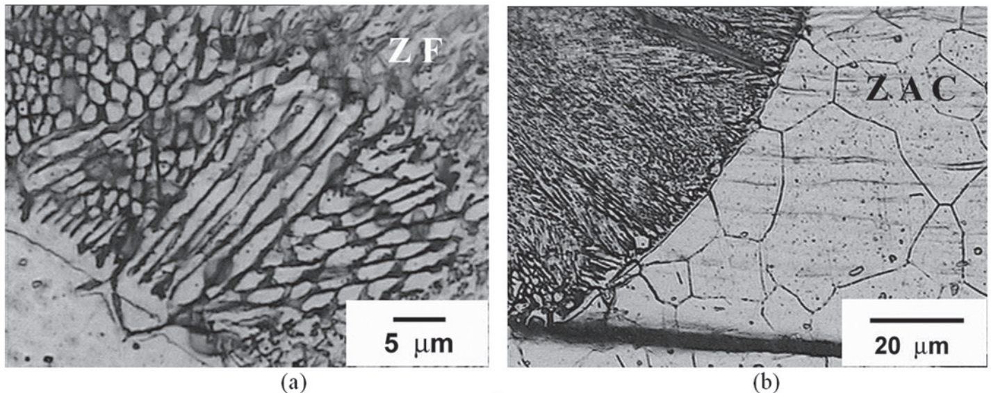
Figura 9. Microestrutura típica da zona de fusão (a) e da ZAC (b) do aço AISI 316L. (amostra soldada com 1,75 Joules).
