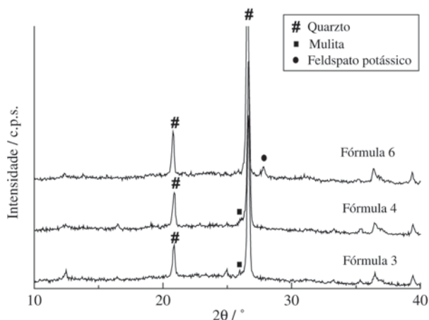
Figura 2. Difratomogramas de raios-X das amostras de Formulações 3, 4 e 6, após a queima.
