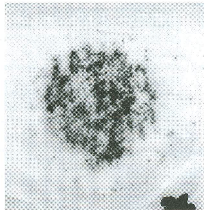
Figura 2. Vista do Depósito de uma Amostra Padrão de Nitrato de Urânio no Makrofol KG após a Contagem na Câmara de Descarga
