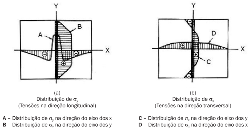
Figura 1 Distribuição esquemática de tensões residuais em uma junta de topo.
