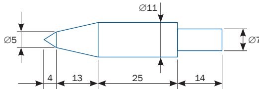
Figura 7 Dimensões da ferramenta.
