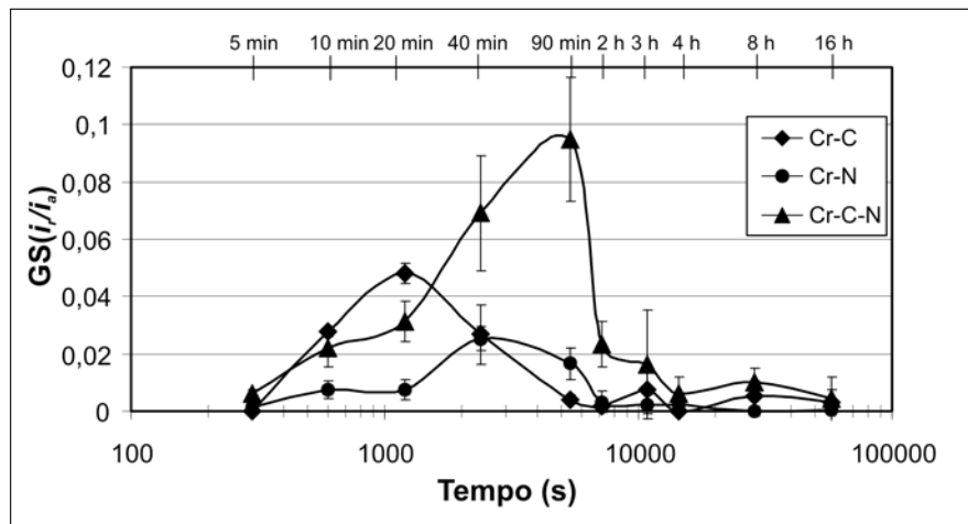
Figura 3 - Variação do grau de sensitização após tratamento isotérmico a 600°C por diferentes tempos para os três aços pesquisados.
