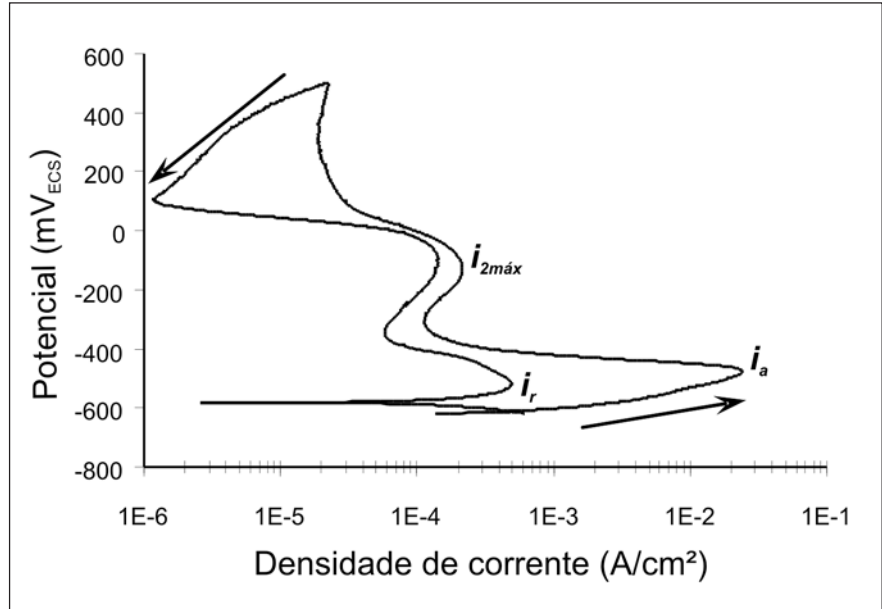
Figura 1 - Curva DL-EPR para o aço Cr-N solubilizado e tratado a 600°C por 40 minutos.
