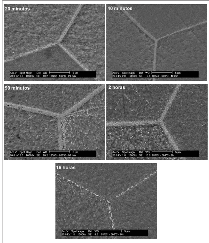
Figura 4 - Precipitados observados em MEV para o aço Cr-N após solubilização e tratamento isotérmico a 600^\circ\text{C} . De 20 minutos a 2 horas, os contornos de grão são totalmente envolvidos pelos precipitados. Em 16 horas, os precipitados são mais grosseiros e mostram descontinuidade (coalescimento).
