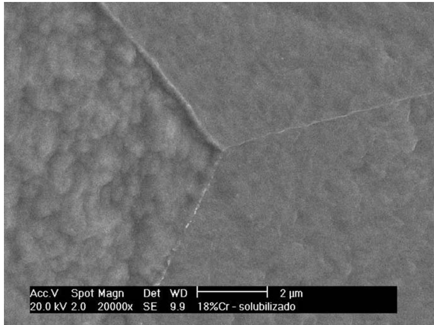
Figura 2 - Micrografia mostrando finos precipitados formados nos contornos de grão ferrítico no aço Cr-N, após tratamento térmico de solubilização. Ataque metalográfico: Vilella. (MEV).
